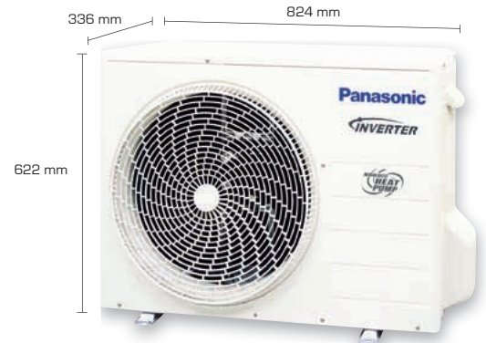
Ulkoyksikkö
